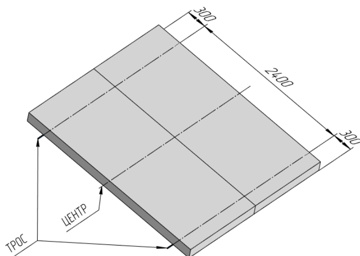
Рисунок 2 – Закладка тросов
